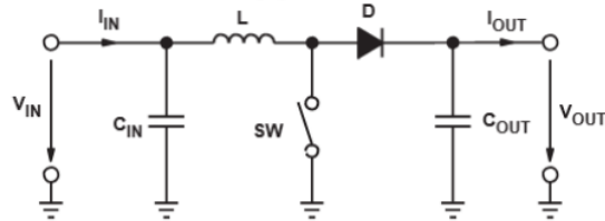
Gambar 2. Rangkaian boost converter secara umum [2].
