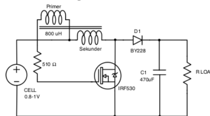
Gambar 4. Sirkuit dari boost converter hasil penelitian
