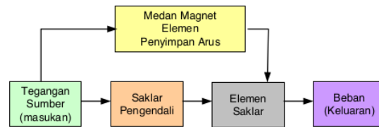
Gambar 3. Diagram blok rangkaian boost converter
