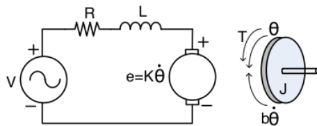
Gambar 4. Persamaan skematik motor DC
