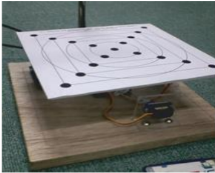
Gambar 7. Ball on plate dilengkapi dengan ball track
