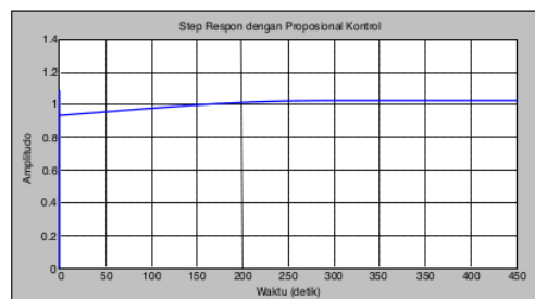
Gambar 11. Hasil Matlab K_p=100 ; K_i=1 ; K_d=1
