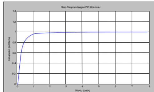
Gambar 13. Step motor respon pada servo motor dengan menggunakan PID kontroler.
