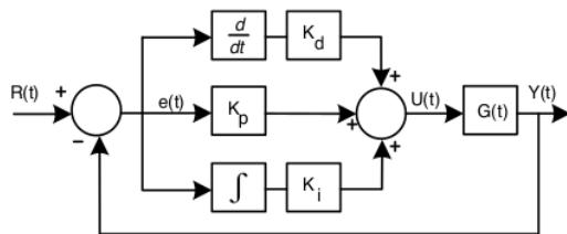
Gambar 3. Kontroler PID
