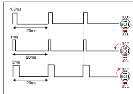
Gambar 2. Sinyal PWM pada servo motor [1].
