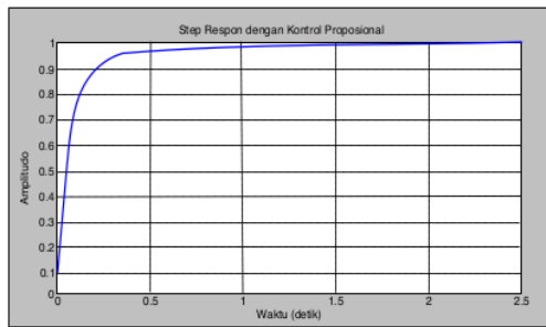
Gambar 12. Hasil Matlab K_p=100 ; K_i=200 ; K_d=10
