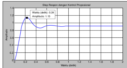
Gambar 10. Hasil Matlab K_p=100 ; K_i=0 ; K_d=0
