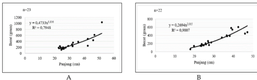
Gambar 6. Korelasi panjang dan berat P. pardalis jantan(A) dan betina (B) di Sungai Ciliwung.
