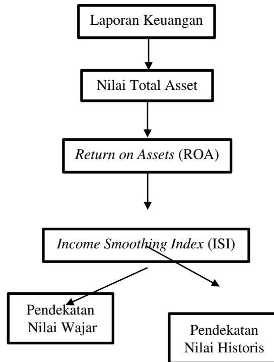
Gambar 1 Kerangka Berpikir
