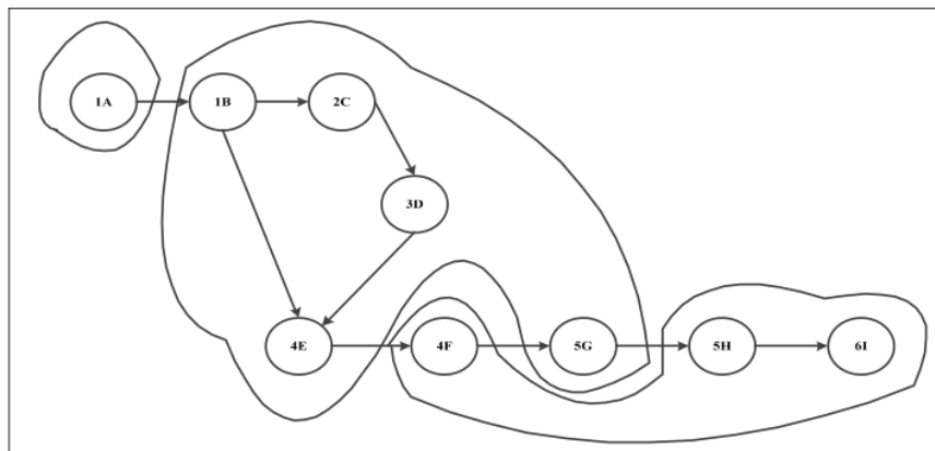
Gambar 6 Usulan Pembagian Stasiun Kerja Pendekatan Metode Wilayah
