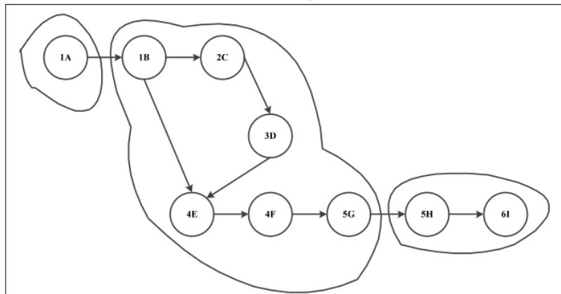
Gambar 7 Usulan Pembagian Stasiun Kerja Pendekatan Pembebanan Berurut
