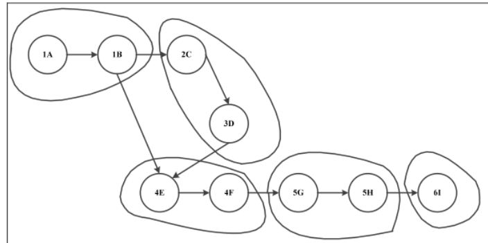
Gambar 3 Pembagian stasiun kerja saat ini
