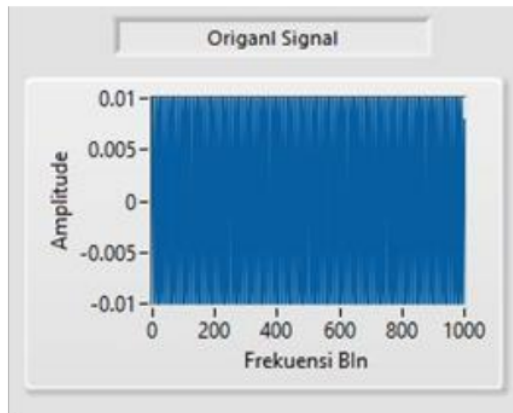
■ Gambar 8. Sinyal Original 100 Hz
