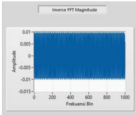
■ Gambar 14. Keluaran Magnitude Sinyal IFFT 150 Hz
