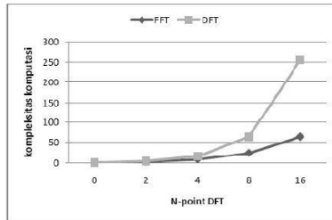
■ Gambar 2. Kompleksitas FFT dan DFT
