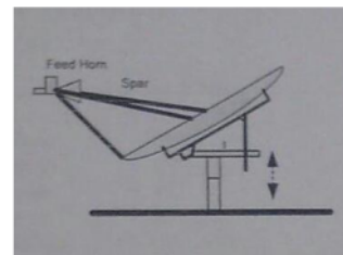
Gambar 8. Bentuk pemasangan spar pada antenna
