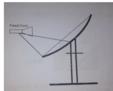
Gambar 4. Bentuk Offset Feed
