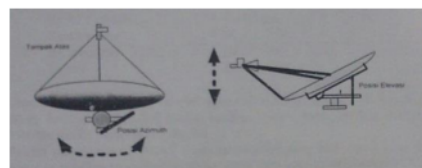
Gambar 9. Posisi azimuth dan posisi elevasi antenna.
