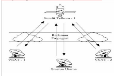
Gambar 2. Komunikasi antar dua VSAT
