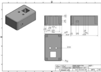
Gambar 7. Desain atas cover
